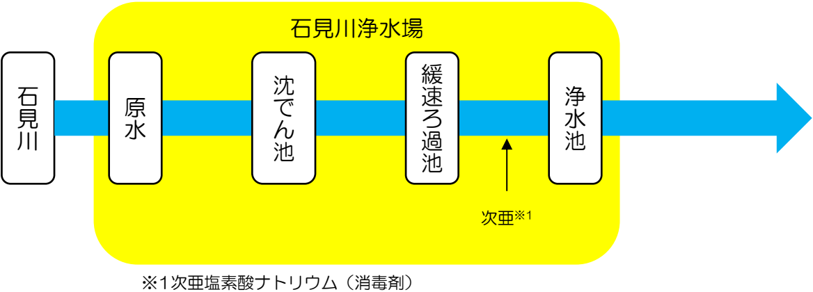
図3 石見川浄水場の処理フロー
