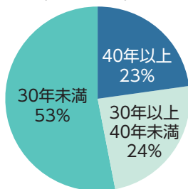
下水道管(汚水)老朽化グラフ(経過年数)
