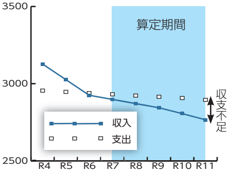
下水道事業の収益的収支見通し(百万円)
