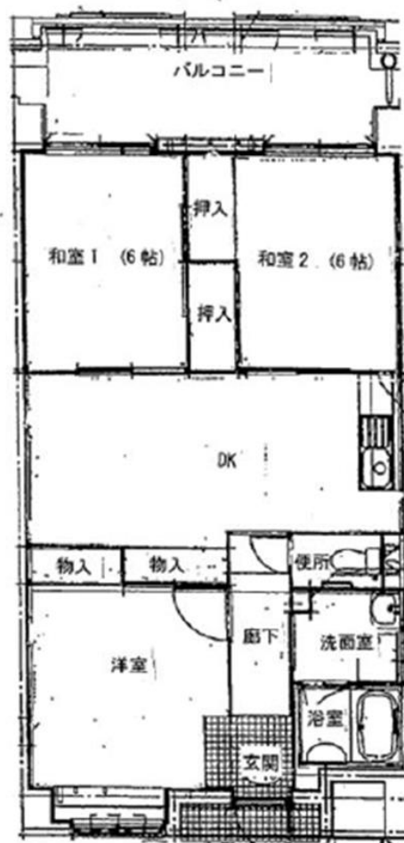
市営三日市西住宅 3DK
