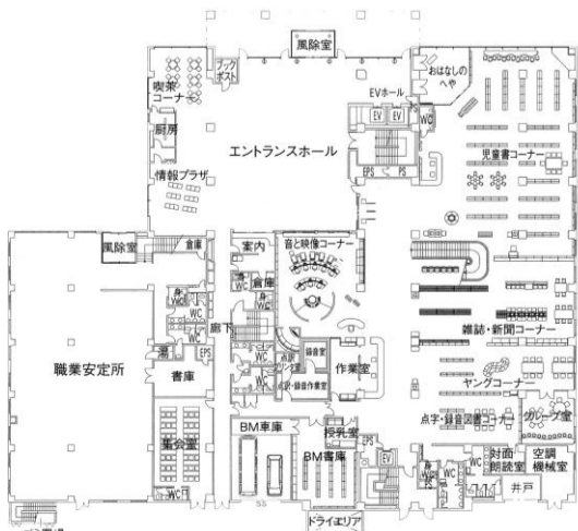
1階平面図
