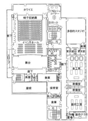
4階平面図
