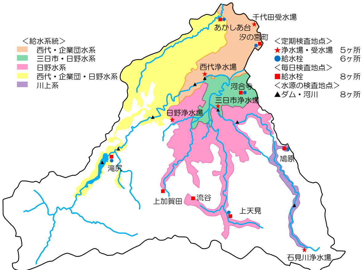
図5 給水区域
